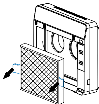
5.2. ábra Szűrő szétszerelése
