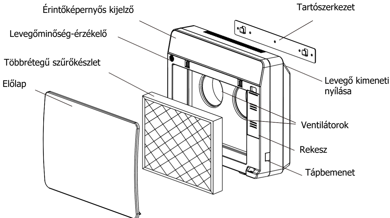
4.1. ábra A készülék részei
