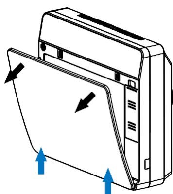
5.1. ábra Előlap leszerelése
